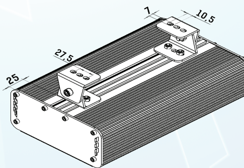
Накладное крепление
